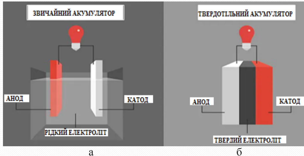
Малюнок 1. Структура літій-іонного акумулятора, структура твердотільного акумулятора
