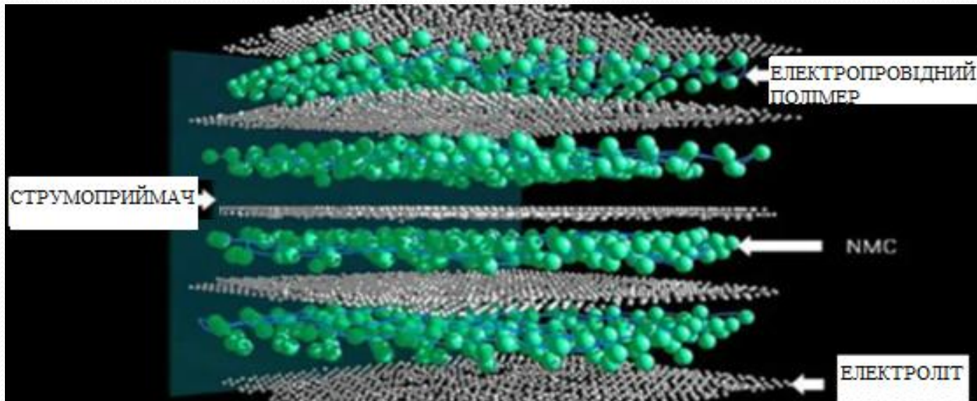
Малюнок 3. Прототип батареї з надтонким керамічним електролітом
