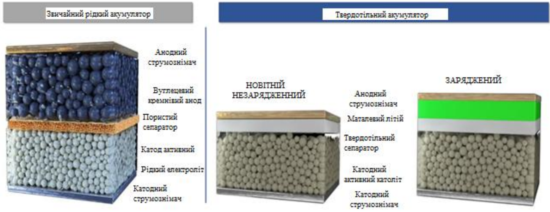
Малюнок 2. Основні шари літій-іонної батареї та батареї з твердотілим електролітом.
