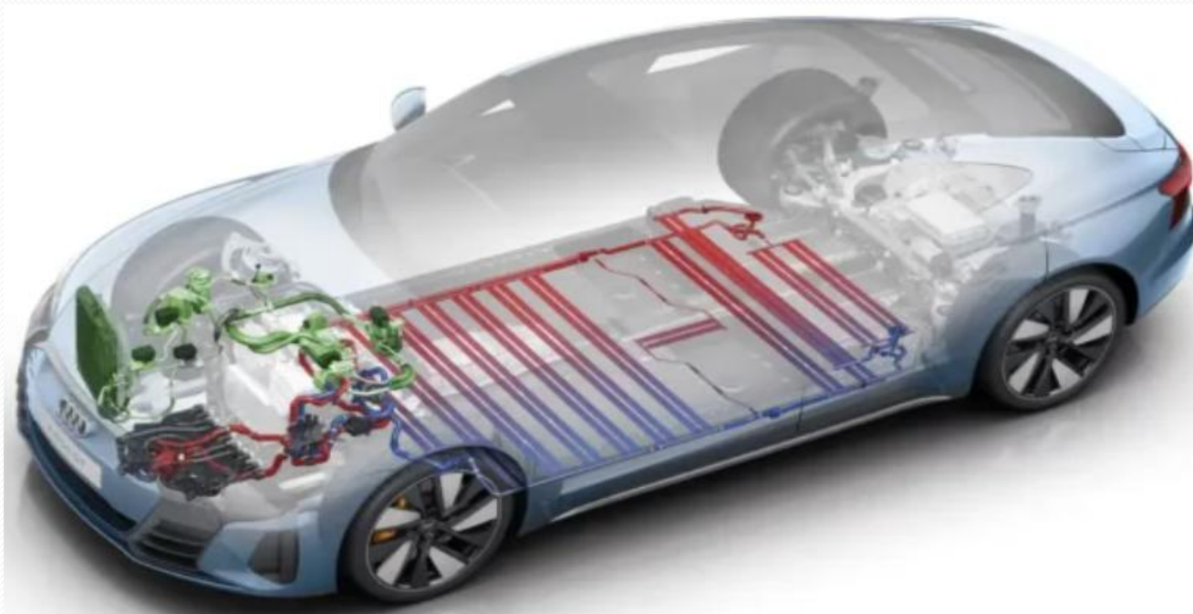
Рисунок 3 - Управління тепловим режимом в електромобілі
