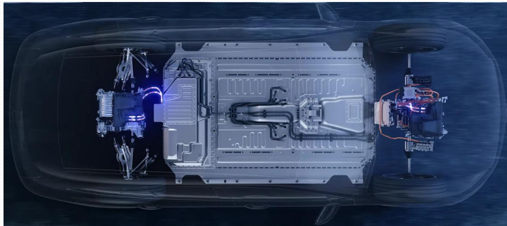
Рисунок 2 – Система охолодження силової електроніки та акумуляторів
