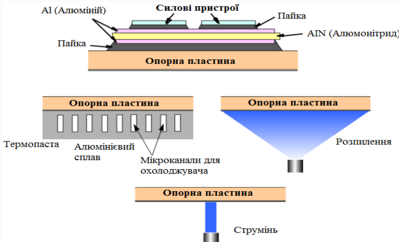
Рисунок 6 – Складова частина системи охолоджувачів
