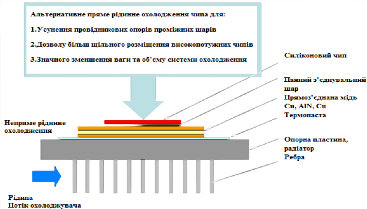
Рисунок 5 - Двофазне охолодження силової електроніки
